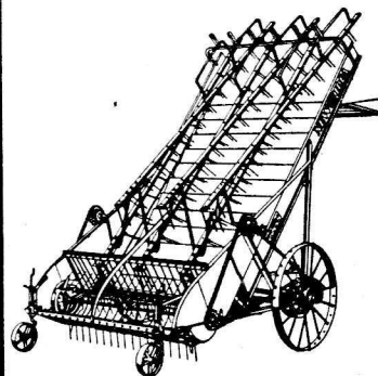
HAY LOADERS
